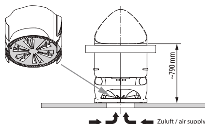
Ofenberührungsschutz optional
