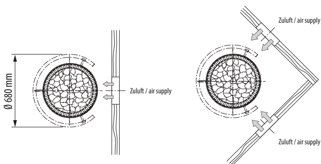
Ofenberührungsschutz optional
