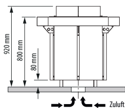
Beispiel für Installation in der Kabinenmitte (Zuluft von unten). Installation vor einer Glas- oder Saunawand (Zuluft seitlich) auch möglich.
