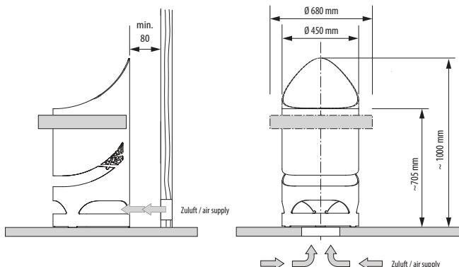
Beispiel für Installation vor einer Glas- oder Saunawand (Zuluft seitlich) / Installation in der Kabinenmitte (Zuluft von unten).
