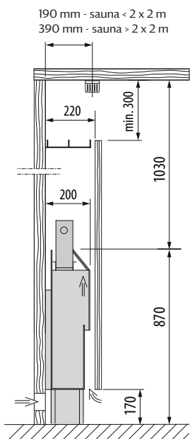
Abb. Verdampfer linksseitig
