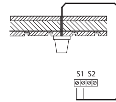
Deckenbefestigung des Fühlers
