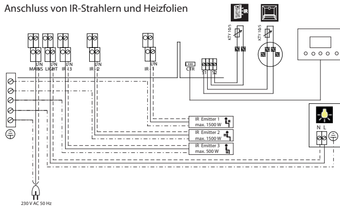
Anschluss von Heizfolien
