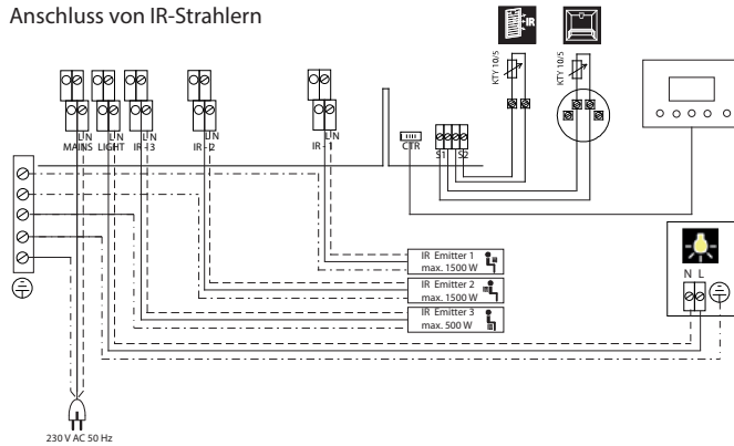
Anschluss von IR-Strahlern und Heizfolien
