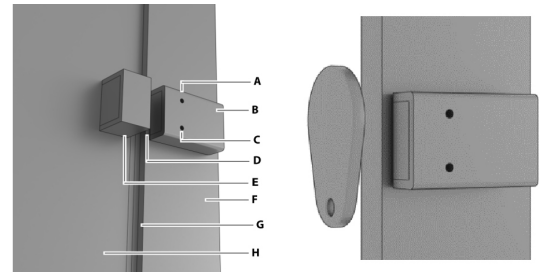
A LED grün D Abstand G Versatz B Türüberwachung E Magnet-Gehäuse H Türblatt J Magnetgehäuse C LED rot F Türrahmen I Magnet K Füllstücke
