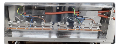
34.G HD:n liitinkotelo: Sisäjohtotuksen suuret kuparikiskot soveltuvat raskaaseen käyttöön.
