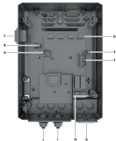
A. RFID-yksikön liitin B. Kaapelin vedonpoisto C. Päävirkakytkin D. Valoverhon liitin E. Kaapelin vedonpoisto F. Väyläyhteyden liitin G. Kaapeliläpivienti valoverholle H. Liitin turvapiirille (STB) I. Kaapeliläpivienti - virtalähteen liitanta J. Kaapeliläpivienti - ohjauskeskuksen liitanta
