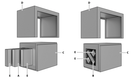
A. Magneetti vertikaalisesti asennettuna B. Magneetti diagonaalisesti asennettuna C. Magneetin koteloointi D. Magneetin kotelon suoja E. Magneetin etäisyydenpitimet
