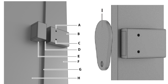
A. LED vihreä B. RFID yksikkö C. LED punainen D. Oviväli E. Ovimagneetti F. Ovikehys G. Oven välyys H. Ovilasi I. RFID-tunniste
