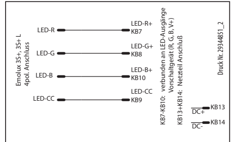
Anschluss an Emolux 3S+, 3S+ L
