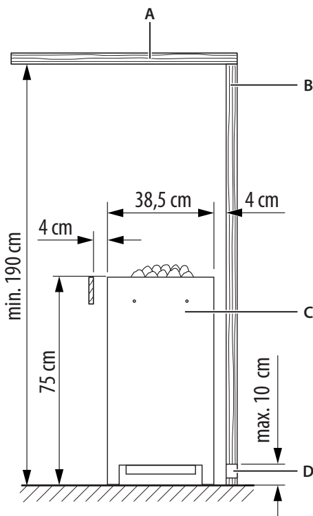
A. Kabinendecke B. Kabinenwand C. Saunaofen
