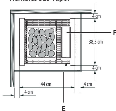
D. Zuluftöffnung E. Ofenschutz F. Verdampferschale (Vapor)
