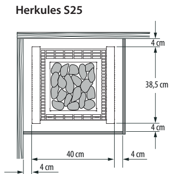
Herkules S25 vapor
