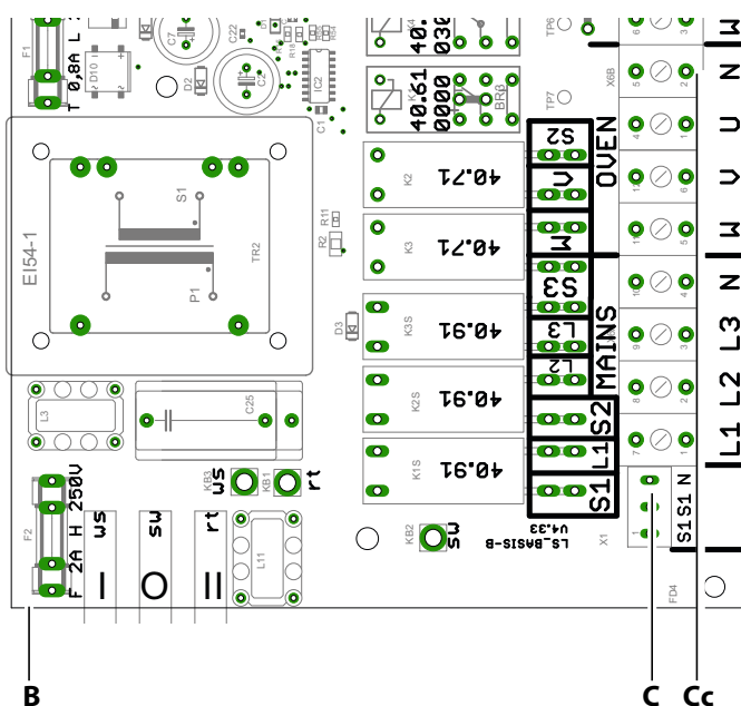
C Anschluss N-Leitung
