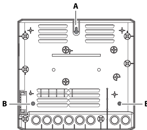
A Oberes Befestigungsloch B Untere Befestigungslöcher
