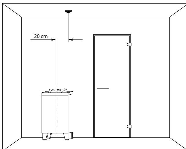
Einbauposition über dem Ofen
