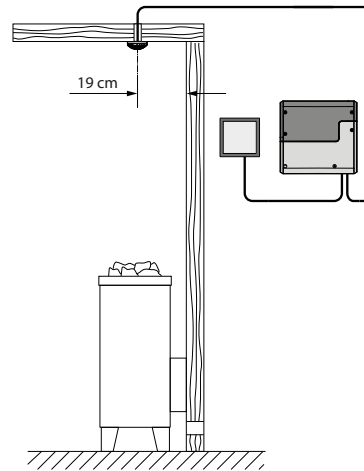
Kabine kleiner 2x2 m
