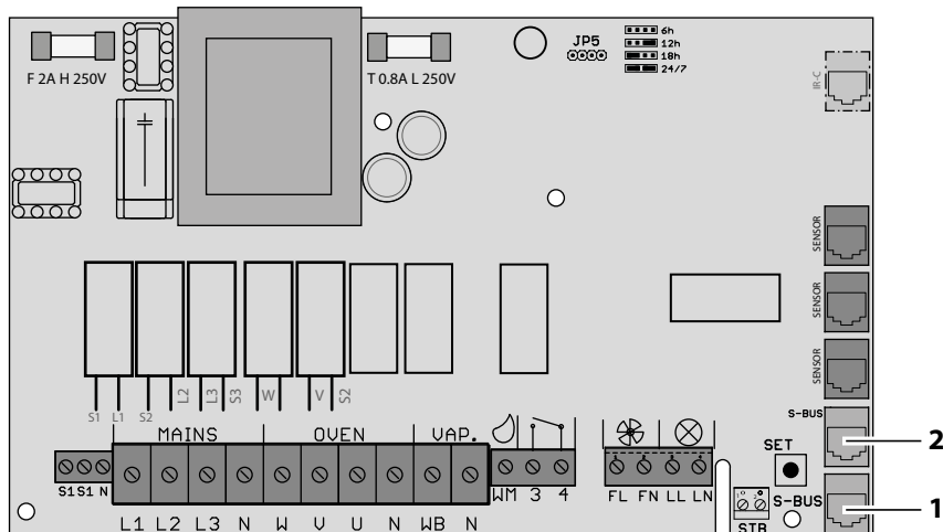
Buchsen – Leistungsteil Saunakabine
