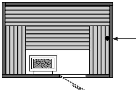
Montageposition Feuchtefühler
