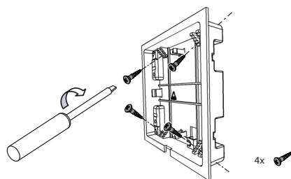
Montage bei Wandstärke > 30 mm
