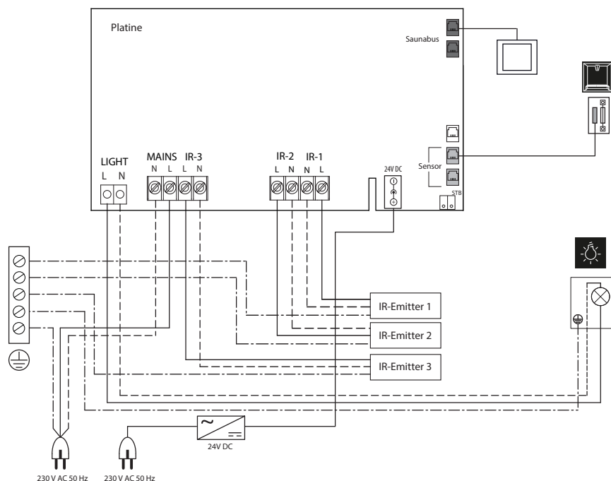
Anschlussbeispiel
