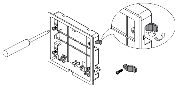
Montage bei Wandstärke 15-30 mm
