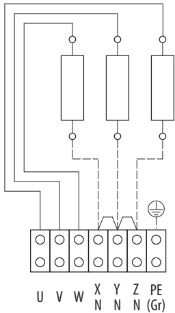
4,5 kW = 3x 1500 W
